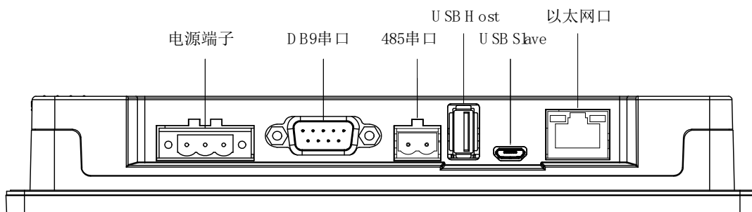
图 4-3 接口图
