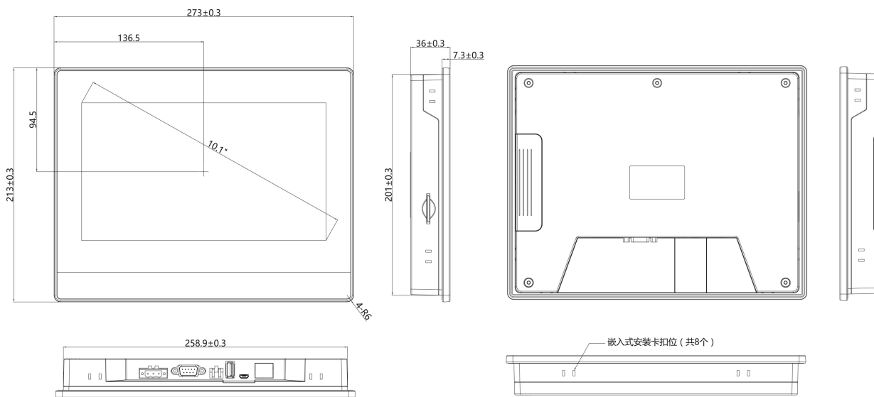
图 6-3 FE6100WE-S01 尺寸图（无 FLink 扩展模块）
