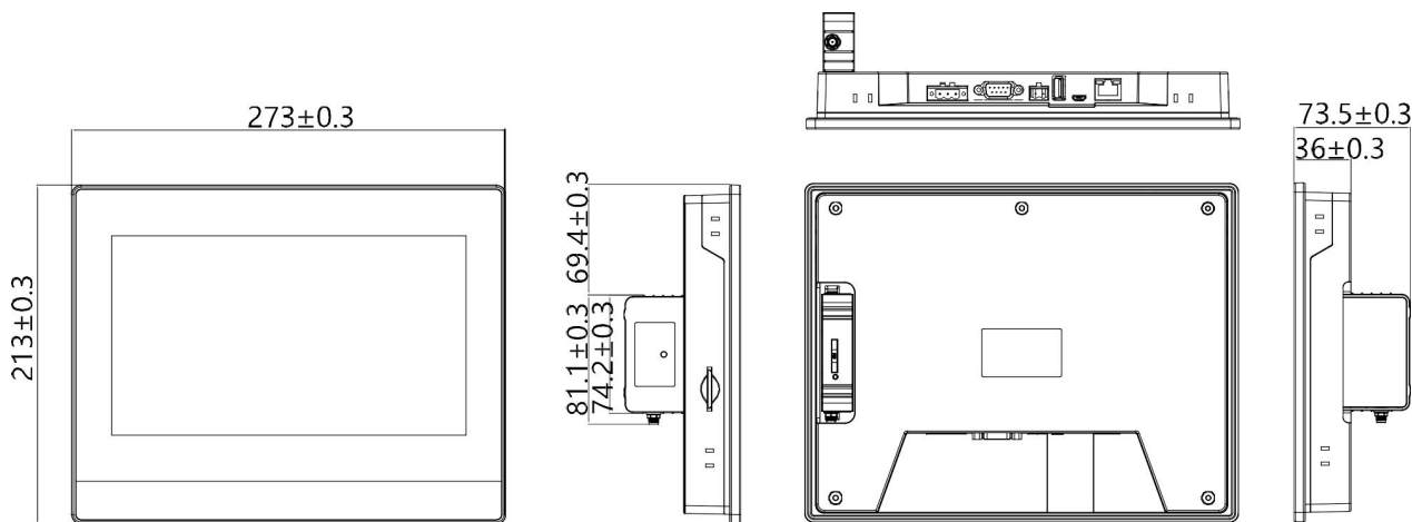
图 6-4 FE6100WE-S01 尺寸图（有 FLink 扩展模块）
