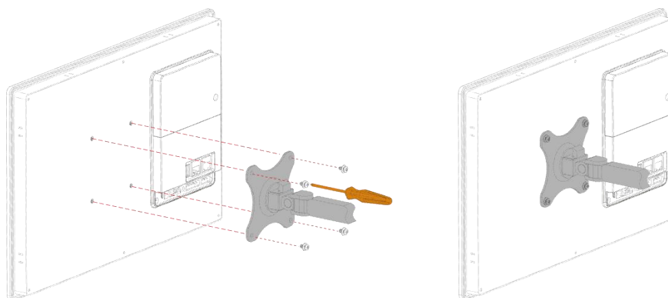
图 5-3 壁挂式安装示意图
