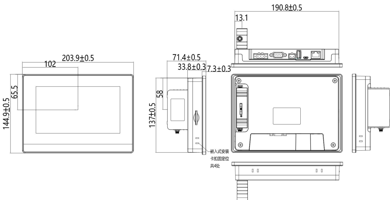
图 6-2 FE6070WE-S01 尺寸图 (有 FLink 扩展模块)
