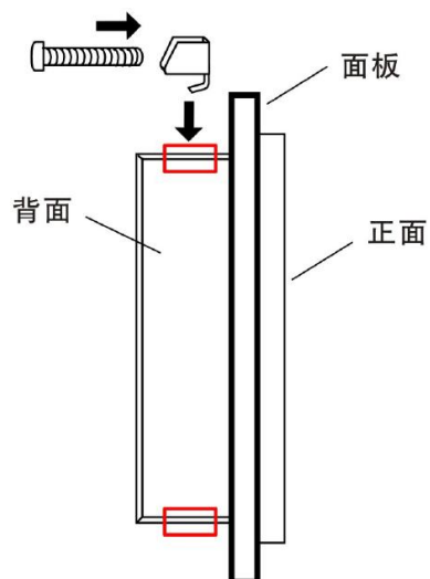
图 5-2 固定触摸屏
