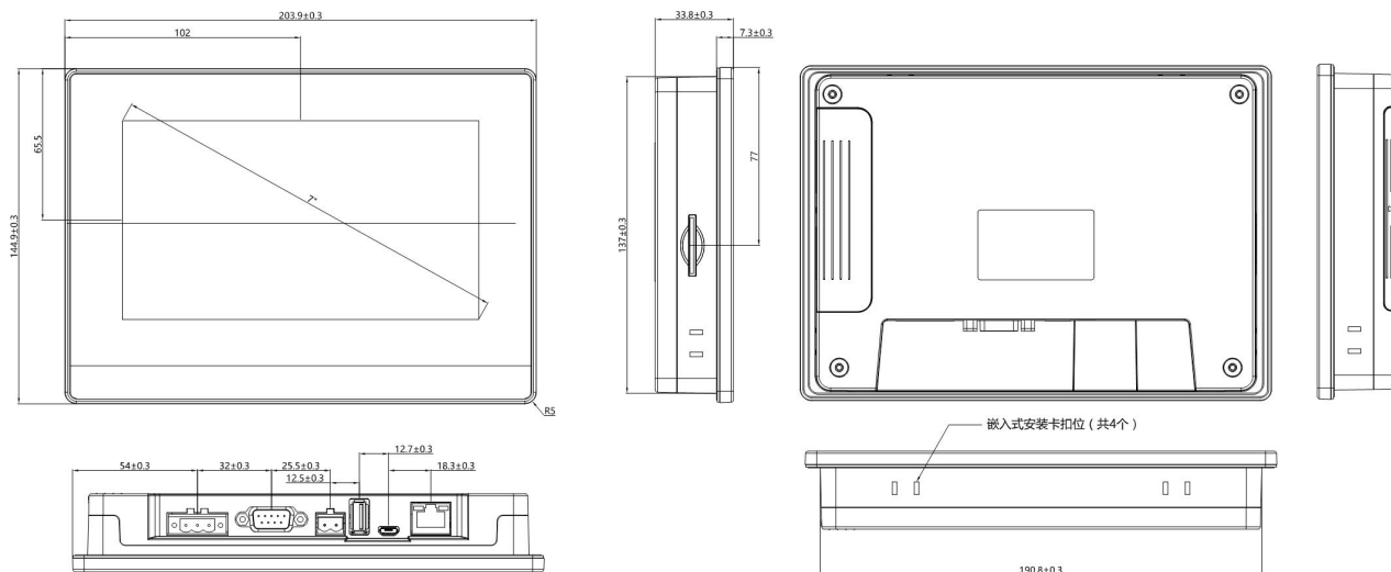
图 6-1 FE6070WE-S01 尺寸图 (无 FLink 扩展模块)
