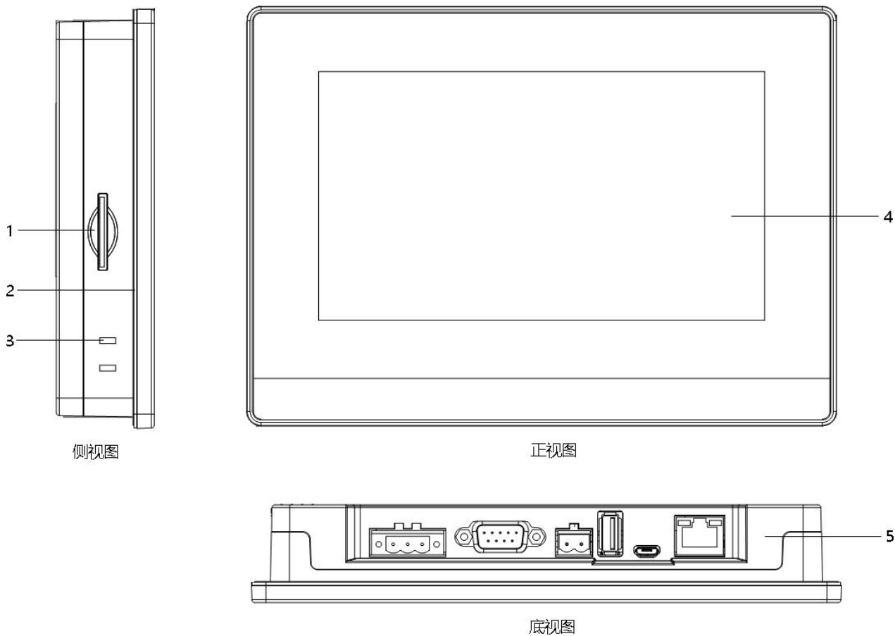
图 4-1 FE6070WE-S01 主视图、侧视图与底视图
