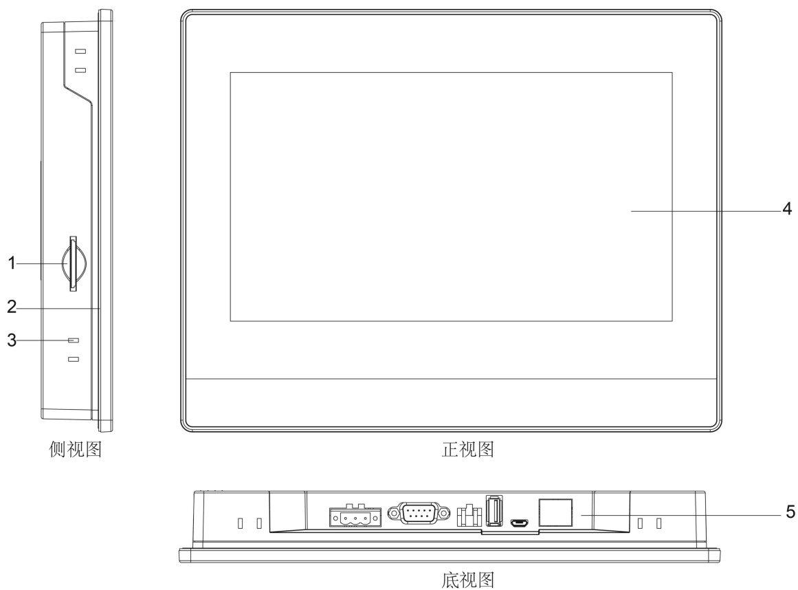
图 4-4 FE6100WE-S01 主视图、侧视图与底视图
