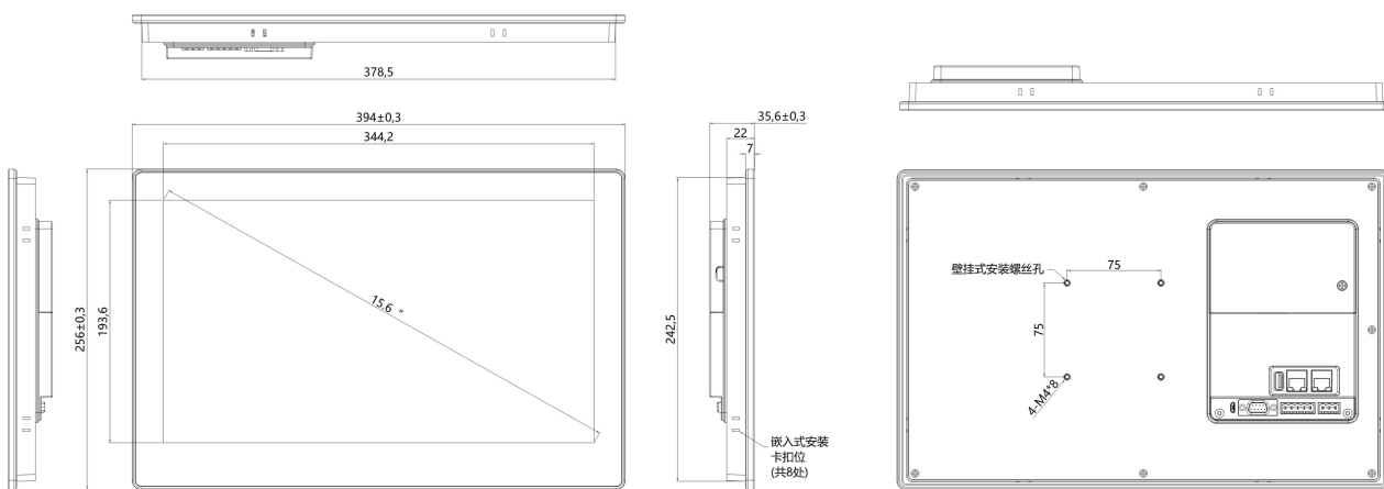
图 6-5 FE6156H-S01 尺寸图
